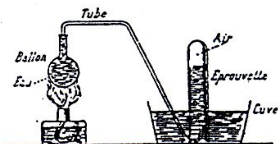
Fig. 1. — Comment on peut recueillir l'air dissous dans l'eau.
